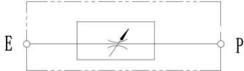
液压原理图
